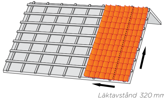
Läggningsskiss
